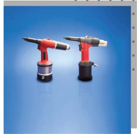
● Pince de pose oléopneumatique pour écrous à sertir
